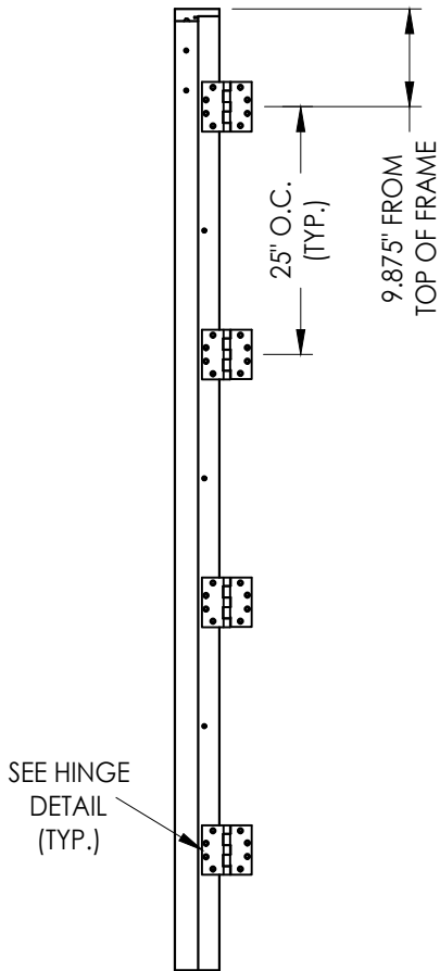
HINGE JAMB
